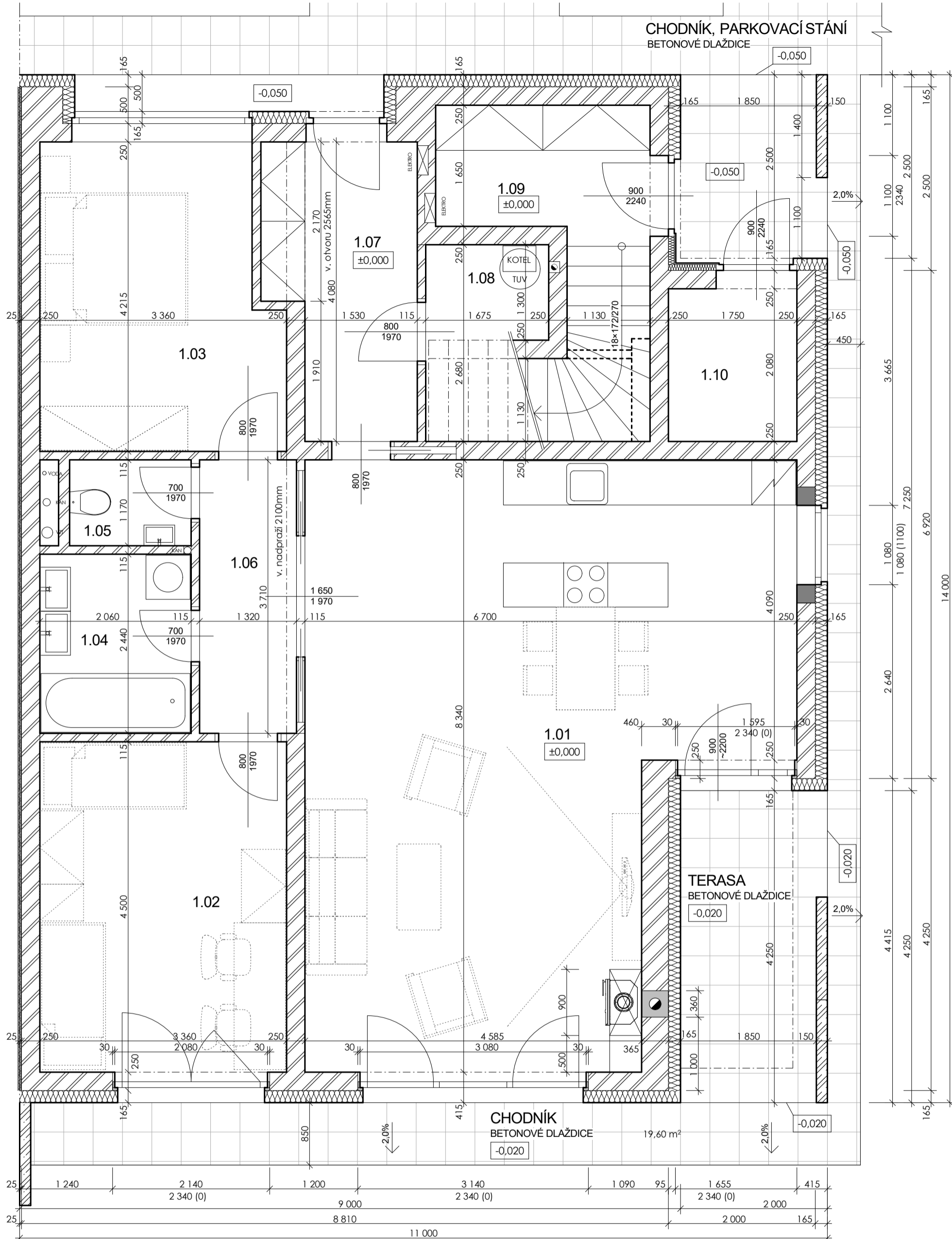
LEGENDA MÍSTNOSTÍ V 1.NP
